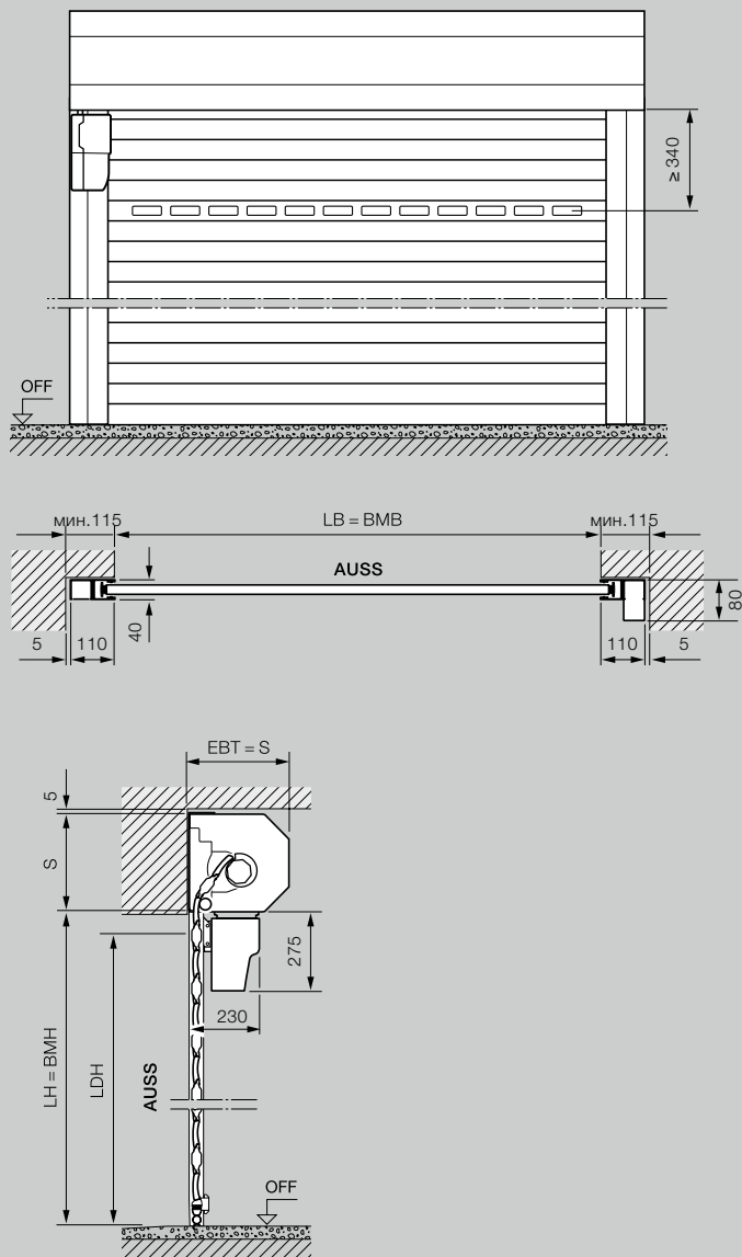
Размери за вътрешна и външна ролетна врата
