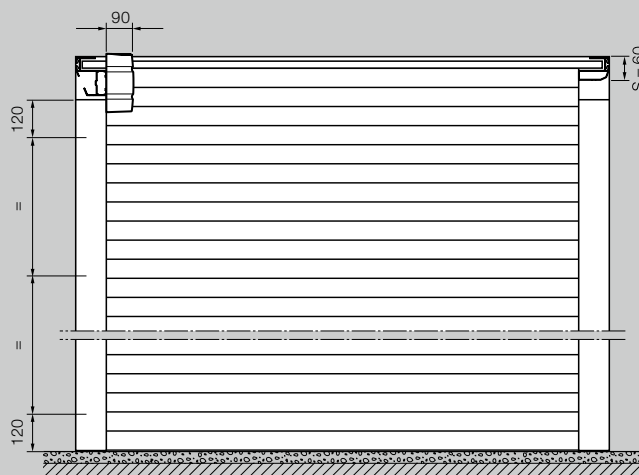
Автоматична врата, прибираща се под тавана Монтаж в отвора, изглед отвътре
